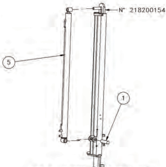
VUE D COLONNE AVANT HYDR. 60"VIEW VIEW D 60" HYDR. FRONT POST
