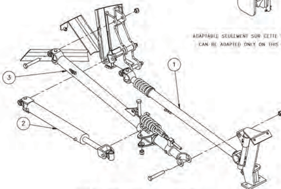
VUE ECLATÉE BRAS DE POUSSE 27" EXPLODED VIEW 27" PUSH ARM
