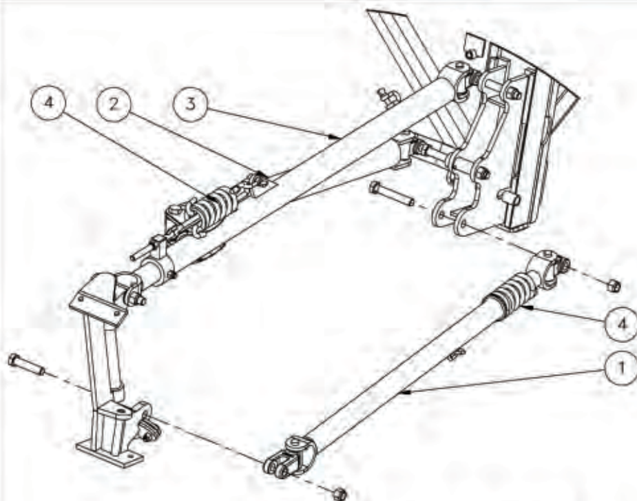
VUE ECLATÉE BRAS DE POUSSE 27" EXPLODED VIEW 27" PUSH ARM
