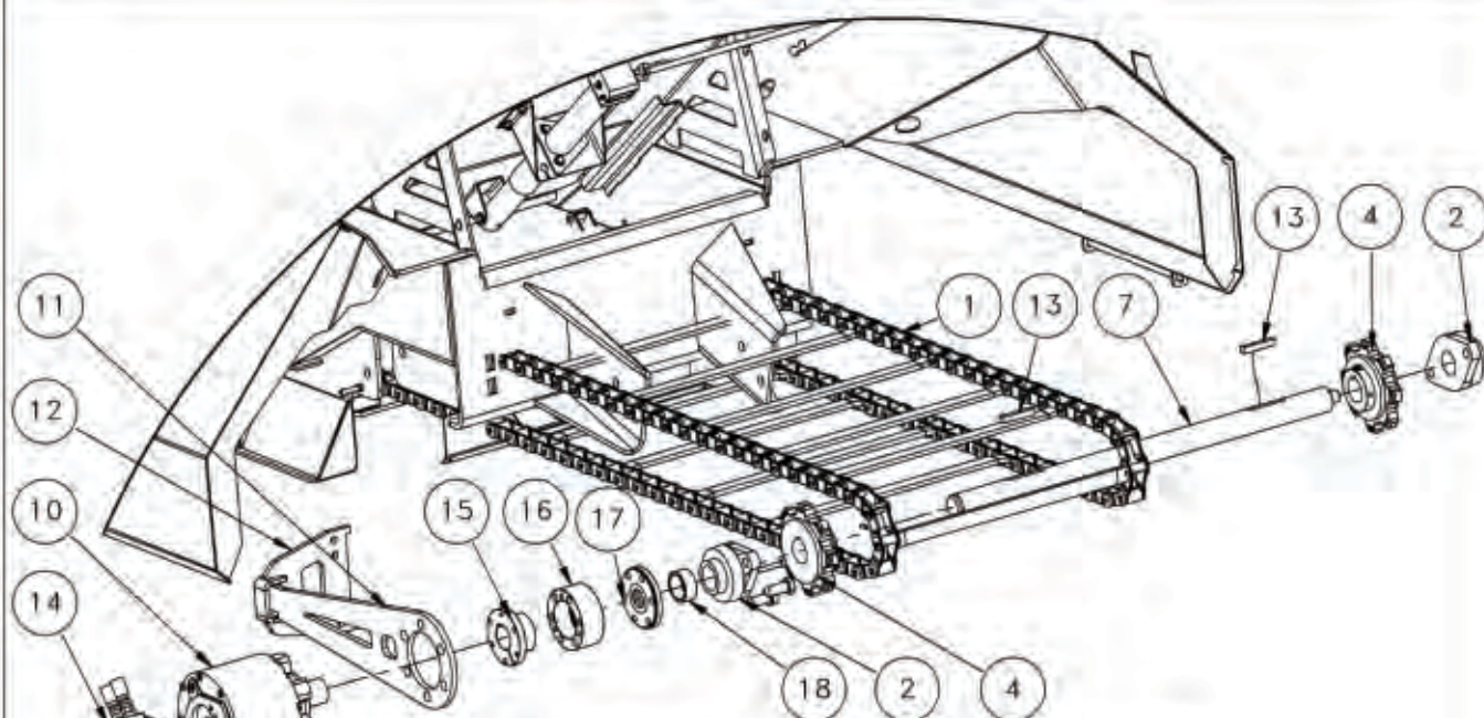
VUE AVANT DE LA CHAÎNE ET DU SYSTÈME MENANT CHAIN FRONT VIEW AND DRIVING SYSTEM
