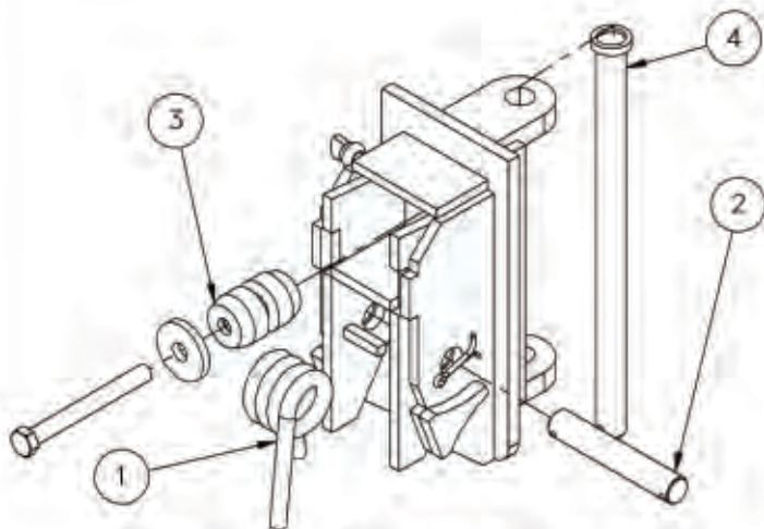
PENTURE 20 DEGRES/20 DEGREE HINGE KIT N° 215220047
