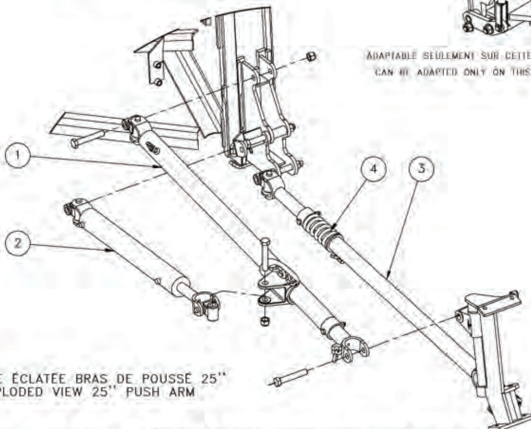
VUE ÉCLATÉE BRAS DE POUSSÉ 25" EXPLODED VIEW 25" PUSH ARM
