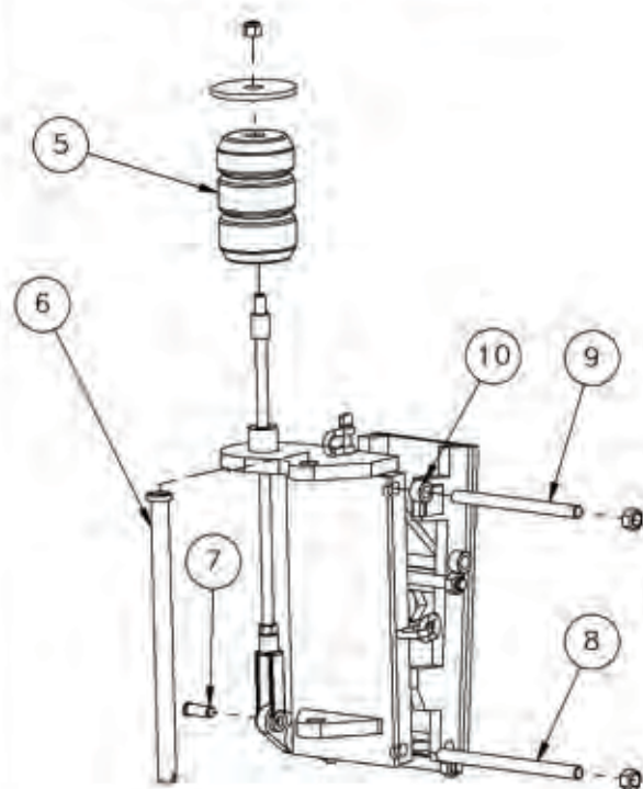
PENTURE 20 DEGRES/20 DEGREE HINGE KIT N° 215220047
